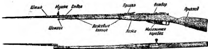
Рис. 1. Общий вид винтовки
