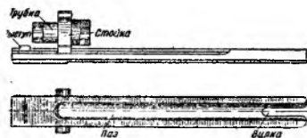
Рис. 10. Соединительная планка
