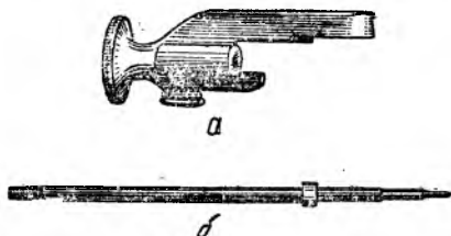
Рис. 6. а — курок, б — ударник
