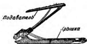
Рис. 12. Крышка магазинной коробки с подающим механизмом
