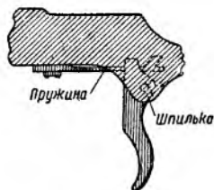
Рис. 16. Спусковой механизм укреплен между ушками ствольной коробки
