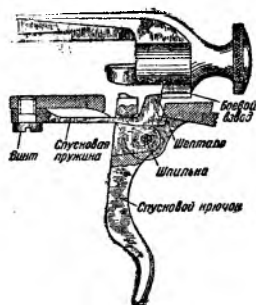
Рис. 8. Шептало заскочило за боевой взвод курка
