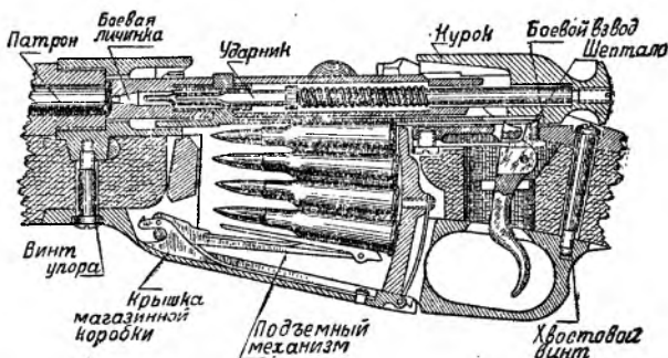
Рис. 5. Разрез винтовки. Положение патронов и частей в заряженной винтовке
