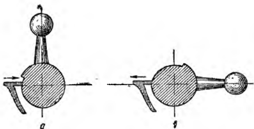
Рис. 14. Рукоятка затвора повернута влево. Лопасть отсечки-отражателя попала в глубокую часть скошенного паза стебля затвора (а). Рукоятка повернута вправо. Лопасть отсечки-отражателя попала в менее глубокую часть скошенного паза стебля затвора и отжалась влево (б)
