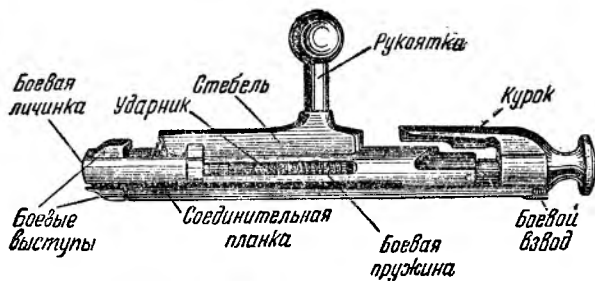
Рис. 2. Затвор в собранном виде
