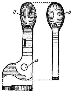
Рис. 78. Рукоять затвора винтовки Карле
