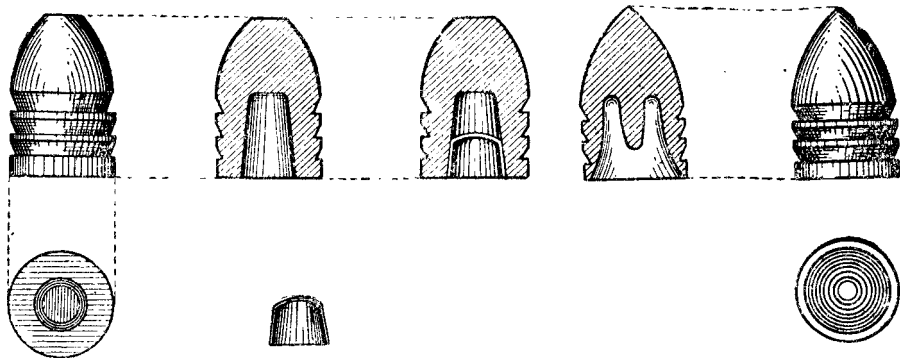
Рис. 62. Пуля Минье
