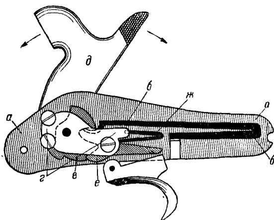
Рис. 49. Ударный замок
