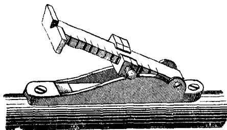
Рис. 134. Прицел секторный с хомутиком
