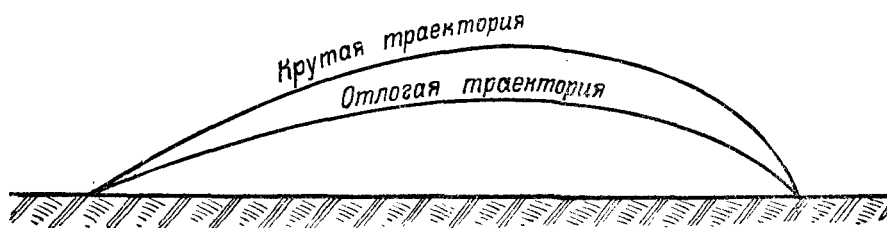
Рис. 32. Отлогая и крутая траектории
