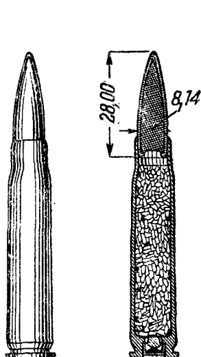
Рис. 124. Германский остроконечный патрон обр. 1904 г.
