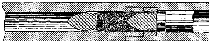
Рис. 70. Двупульная система Жилле-Грина
