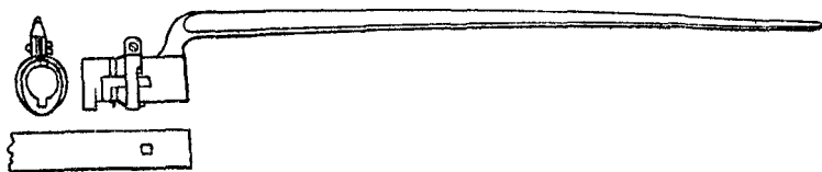
Рис. 31. Штык с шейкой
