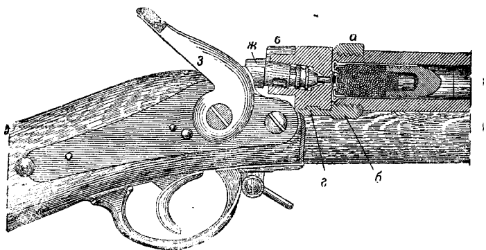
Рис. 96. Продольный разрез казенной части винтовки Крюка
