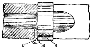
Рис. 97. Схема действия выбрасывателя винтовки Крюка — затвор закрыт
