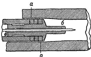
Рис. 73. Обтюратор винтовки Шасспо
