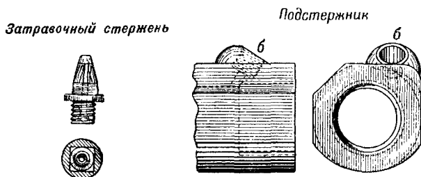
Рис. 48. Подстержник и затравочный стержень ударного ружья
