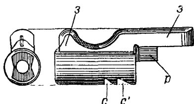
Рис. 115. Курок винтовки Гра обр. 1874 г.
