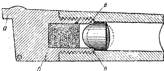
Рис. 54. Казенная часть штуцера Дельвиня
