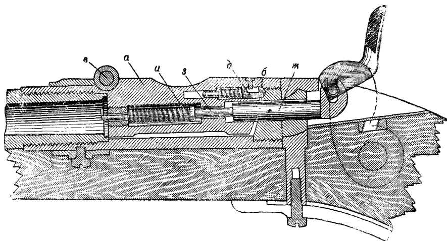
Рис. 91. Винтовка системы Альбини-Баранова — продольный разрез
