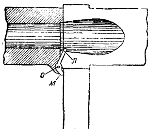
Рис. 98. Схема действия выбрасывателя винтовки Крюка — затвор открыт
