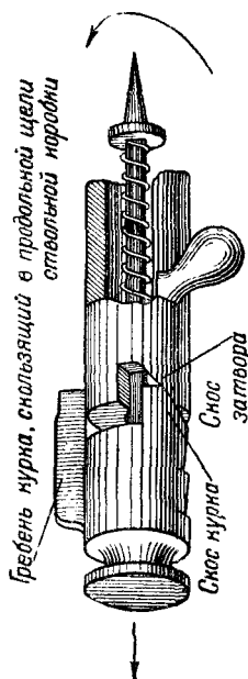
Рис. 113. Введение курка помощью винтовых ско- сов на курке и стебле затвора
