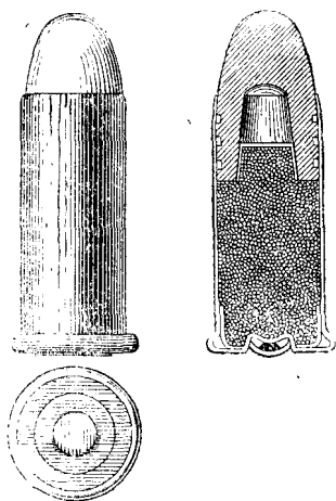
Рис. 99. Патрон к винтовке Крюка
