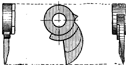
Рис. 103. Выбрасыватель винтовки Бердана № 1
