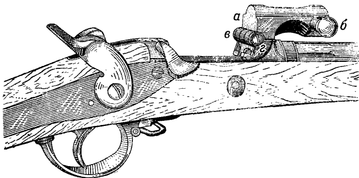
Рис. 90. Винтовка системы Альбини-Баранова — затвор открыт
